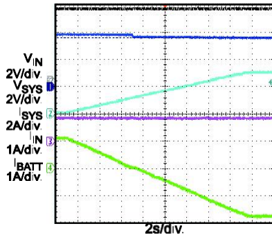
Input Current Limit USB3.0 Mode, V_{BATT} = 3.7V Ramp up I_{SYS}
