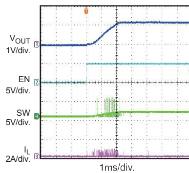
EN Start Up without Load
