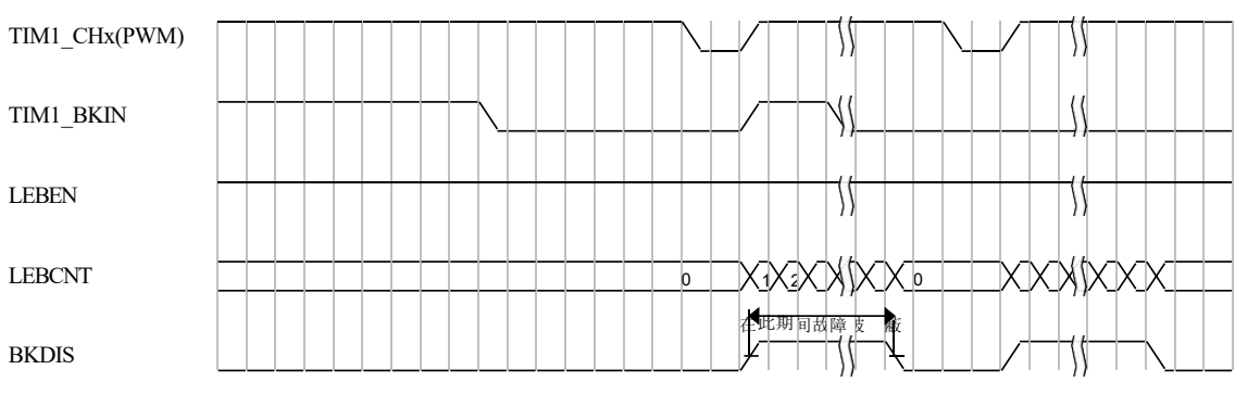
图 10.41 前沿消隐时序示意图
