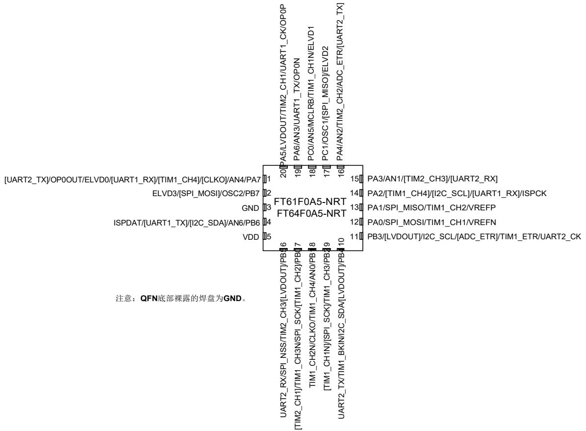
图 1.6 QFN20 脚位
