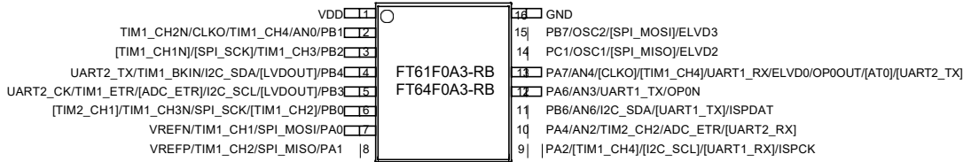
图 1.4 SOP16 脚位
