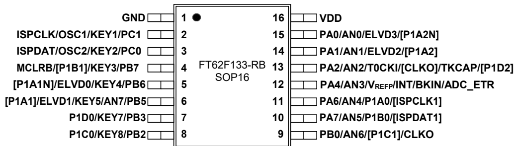
图 1-5 SOP16 1
