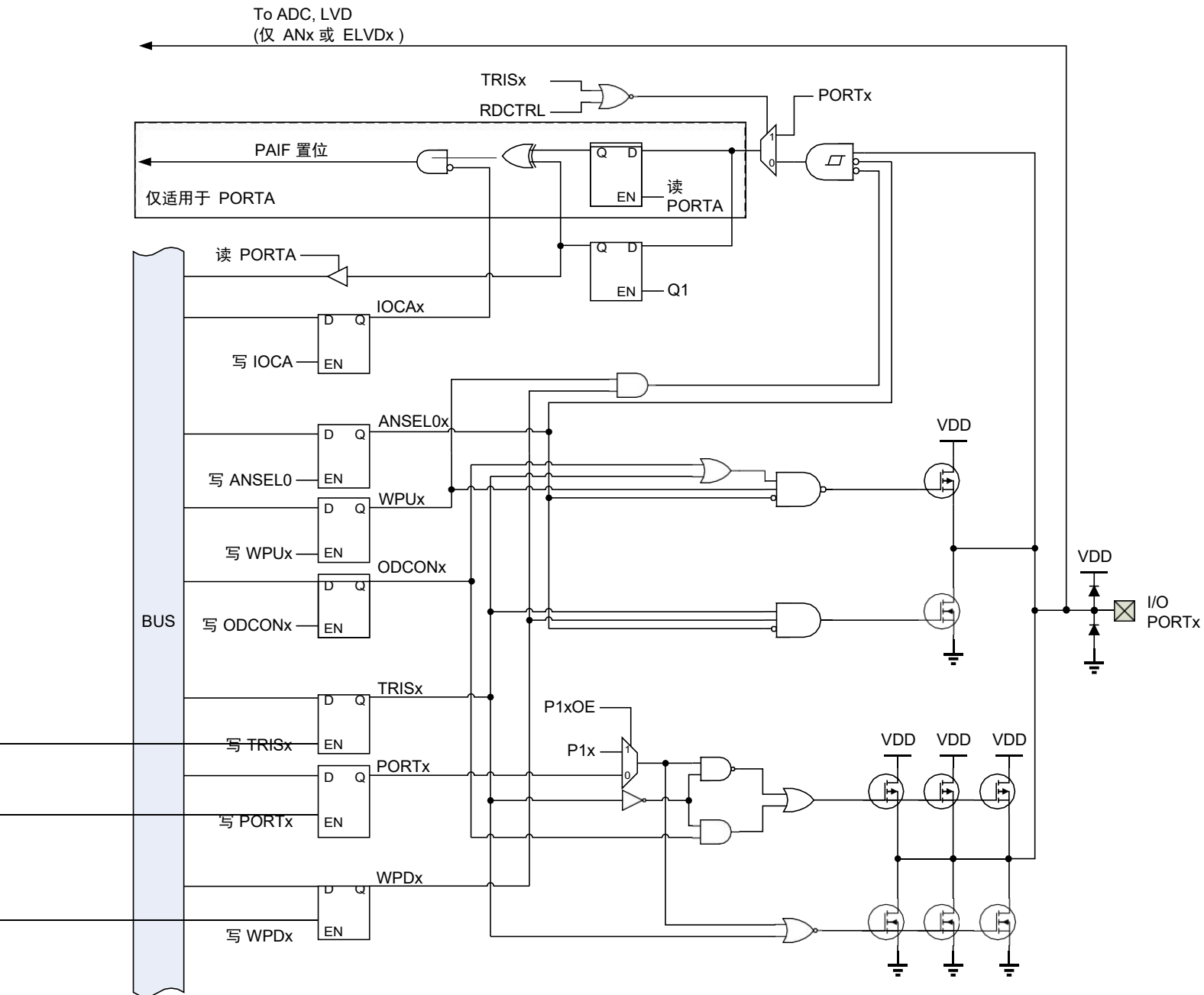
图 2-1 PORT 端口结构框图
