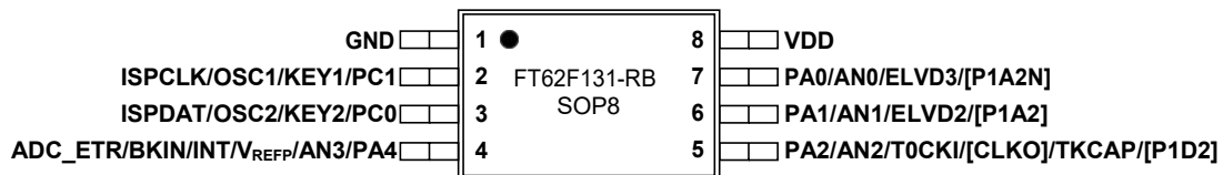
图 1-2 SOP8 1
