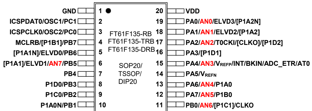
图 1.6 SOP20/TSSOP20/DIP20 脚位
