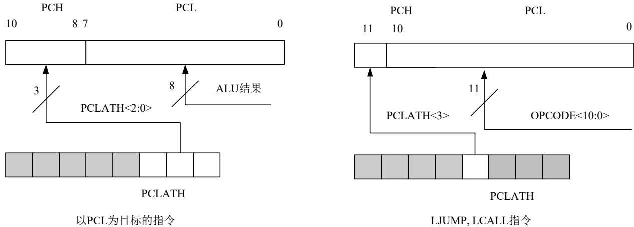
图 2.1 不同情况下 PC 的加载
