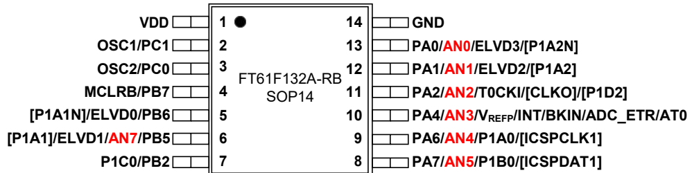
图 1.4 SOP14 脚位
