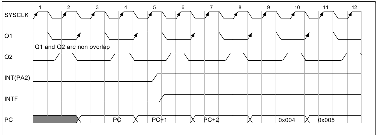
图 6.3 中断响应时序图
