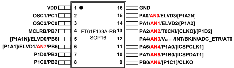
图 1.5 SOP16 脚位
