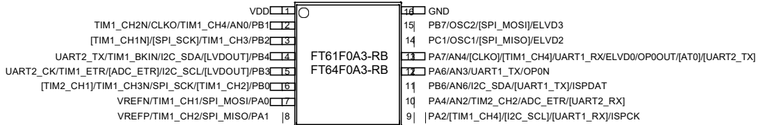
图 1.4 SOP16 脚位
