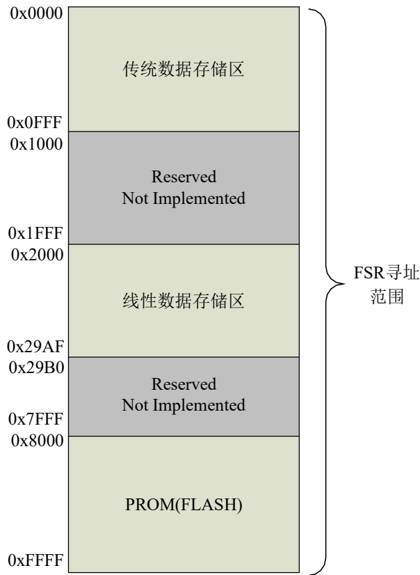
图 3.4 间接寻址
