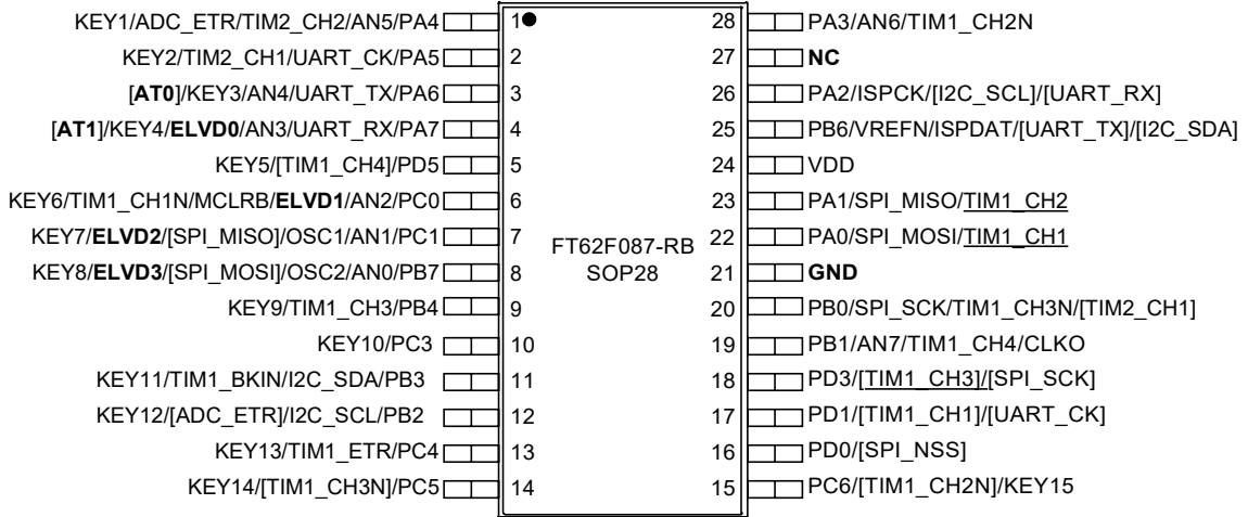
图 1.5 SOP28 脚位
