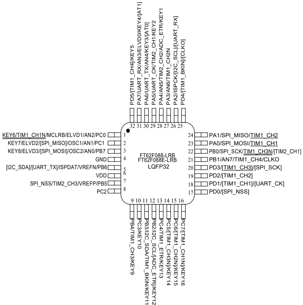
图 1.6 LQFP32 脚位
