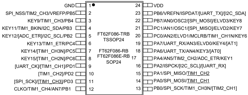
图 1.4 SOP24/TSSOP24 脚位
