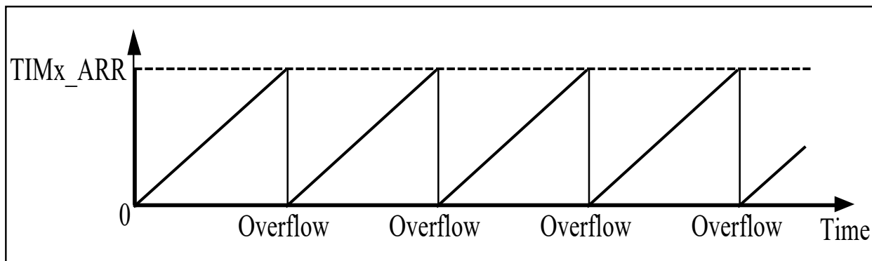
图 11.3 向上计数器
