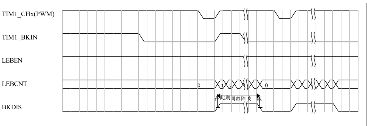
图 10.41 前沿消隐时序示意图
