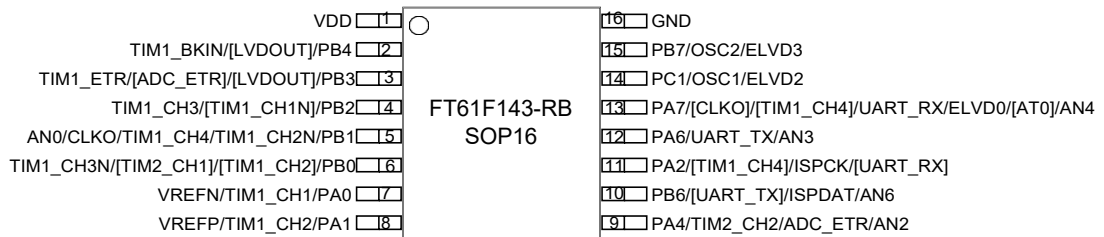
图 1.6 SOP16 脚位
